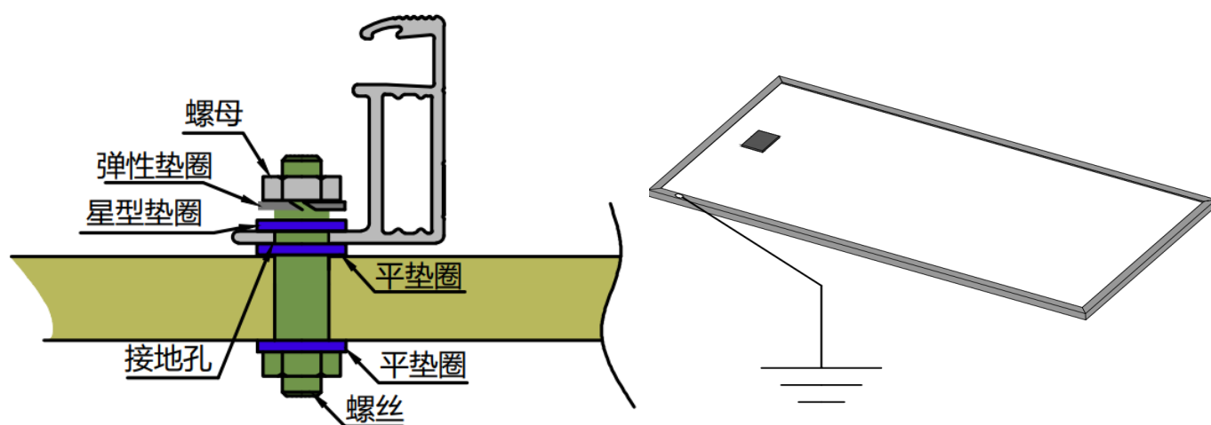
图11 组件接地图
