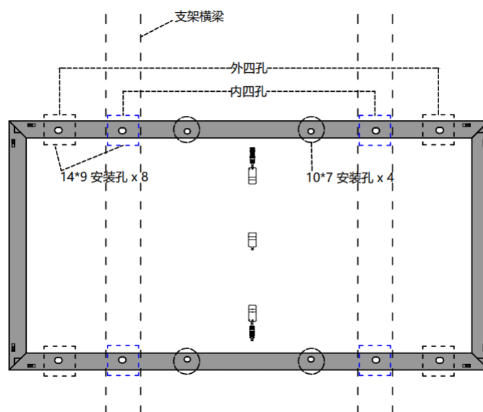
图3 螺栓安装的方式（内4孔）
