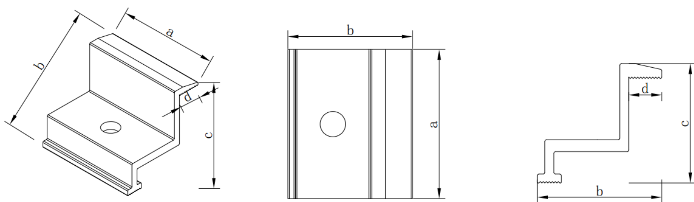
图 4 压块
